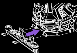
Instalar Limpiacharcos (4 tornillos)
